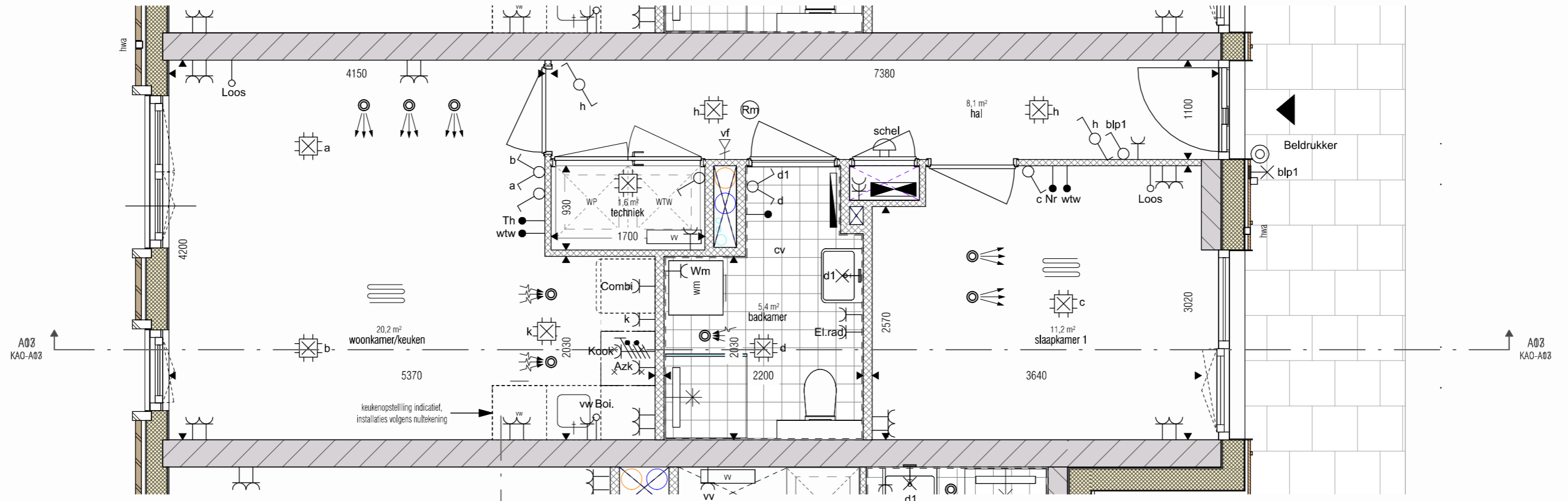
KAO_BNR A03_00 begane grond 1 : 50
