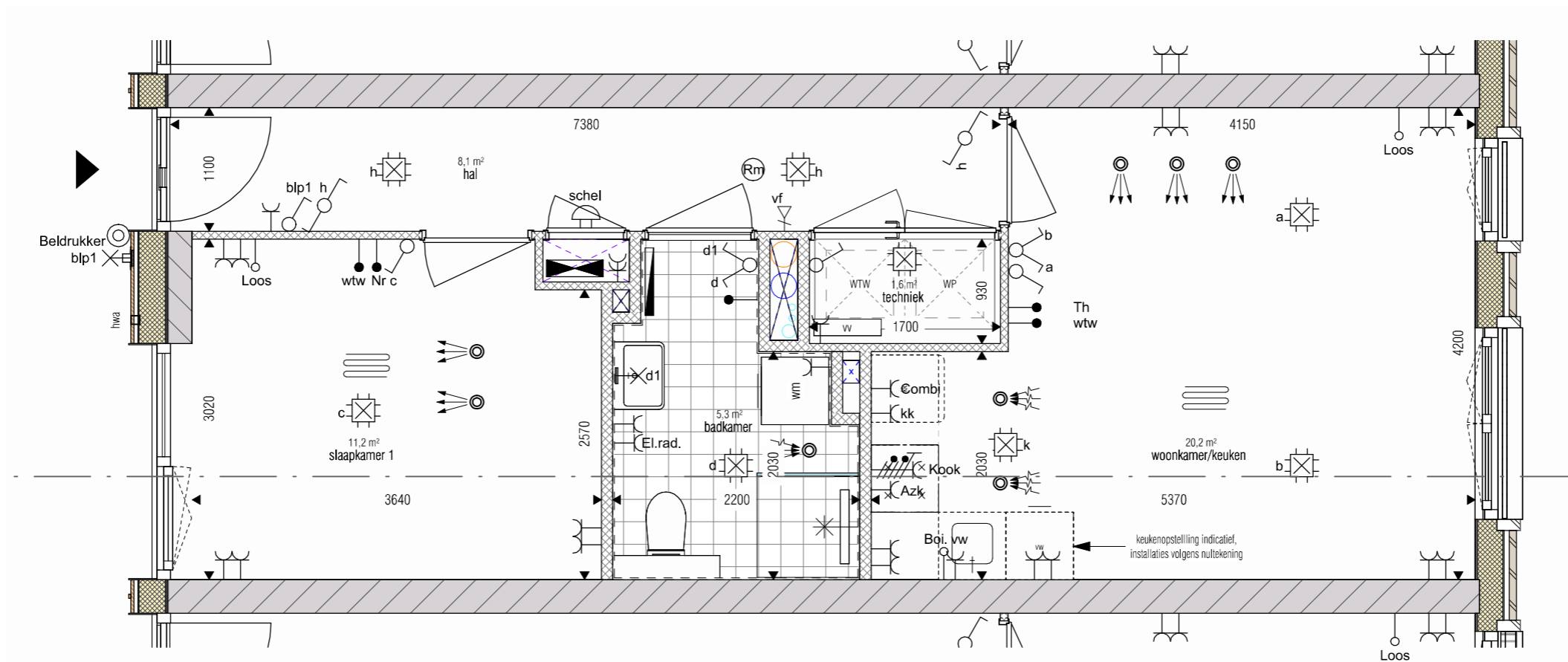
BNR A29_01 eerste verdieping 1 : 50
