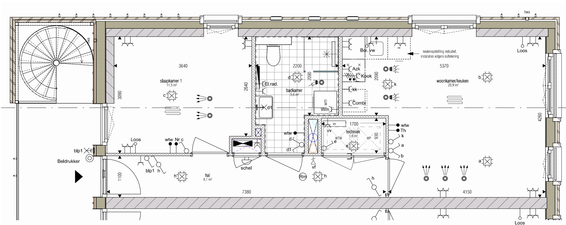
BNR A30_01 eerste verdieping 1:50
