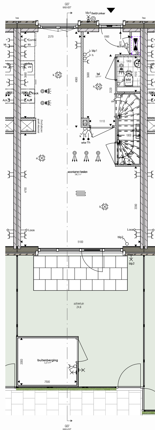
BNR G07_00 begane grond 1:100
